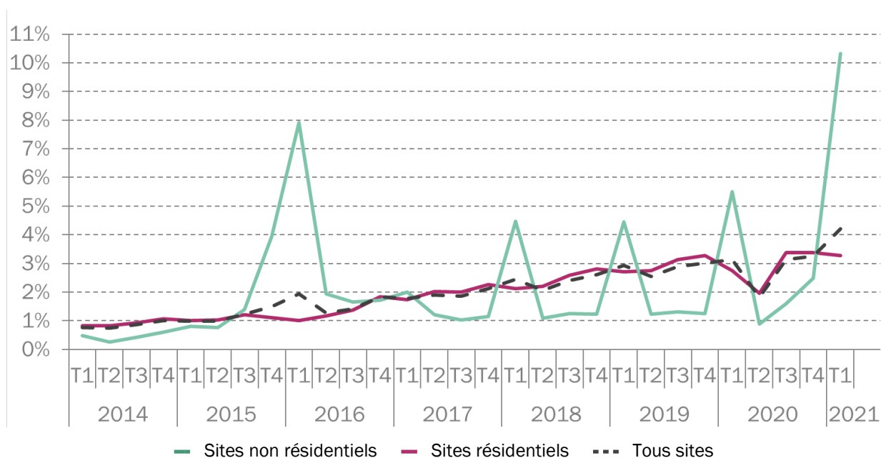
Figure 14 : Évolution du taux de switch par segment de clientèle
